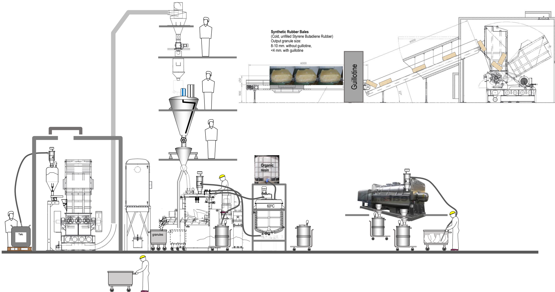
СХЕМА ИЗМЕЛЬЧЕНИЯ ТЮК СИНТЕТИЧЕСКОГО КАУЧУКА, ПЕРЕМЕШИВАНИЯ И ГРАНУЛИРОВАНИЯ КОМПОНЕНТОВ ДЛЯ ПРОИЗВОДСТВА РЕЗИНОТЕХНИЧЕСКИХ ИЗДЕЛИЙ
